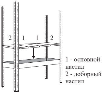
Рис. 5 а Укладка металлического настила
