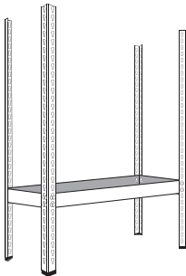
Рис. 6 а Вид стеллажа без настила под шины
