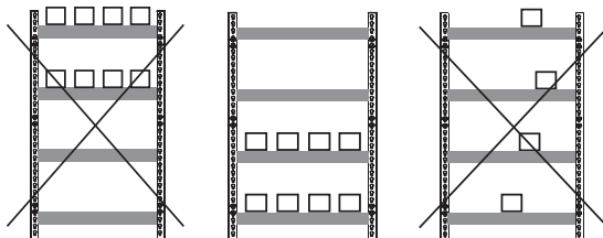
Схема распределения нагрузки
